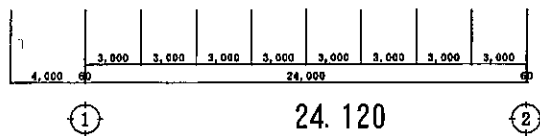
平面図 S 1:200
