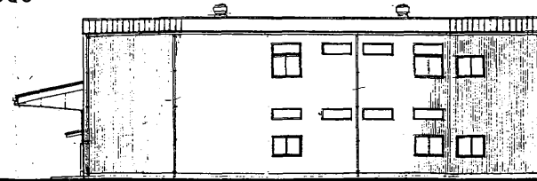
東立面図
