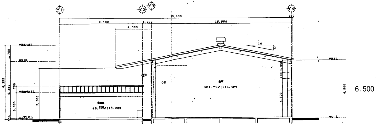
X-X 断面图
