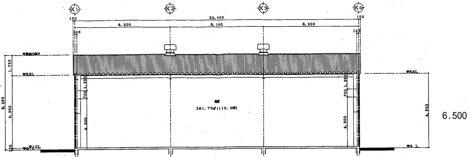
X-X 断面图
