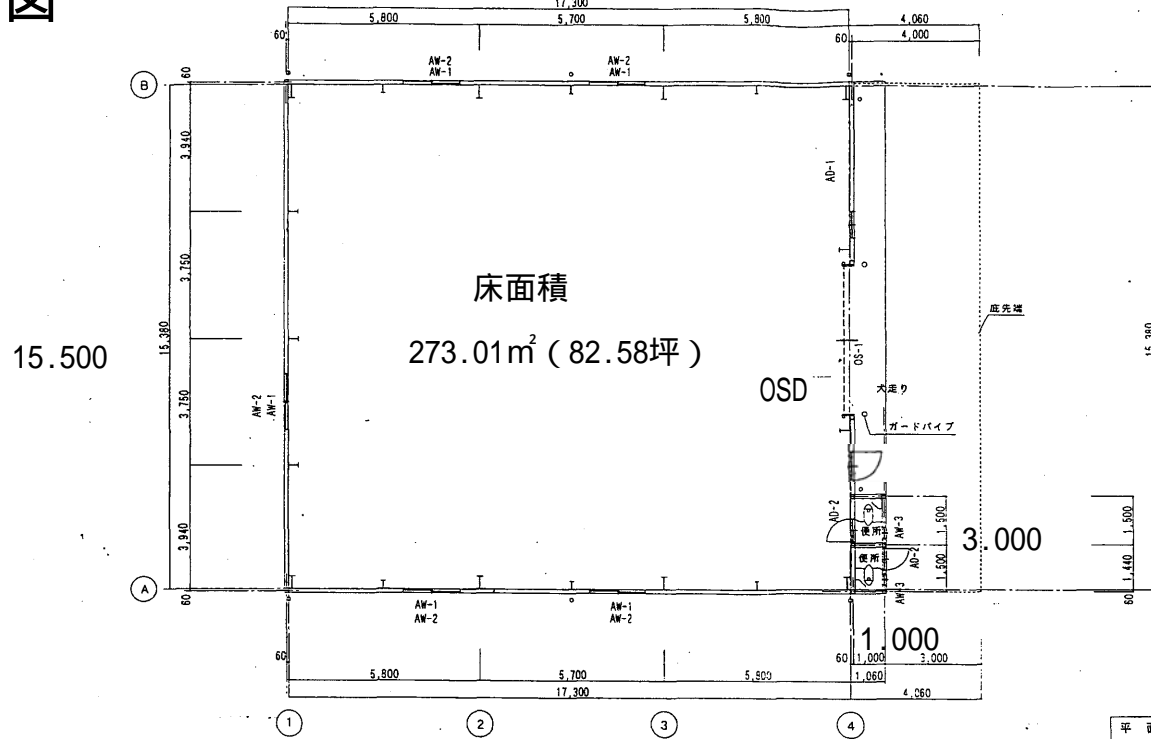
平面図 S=1/100
